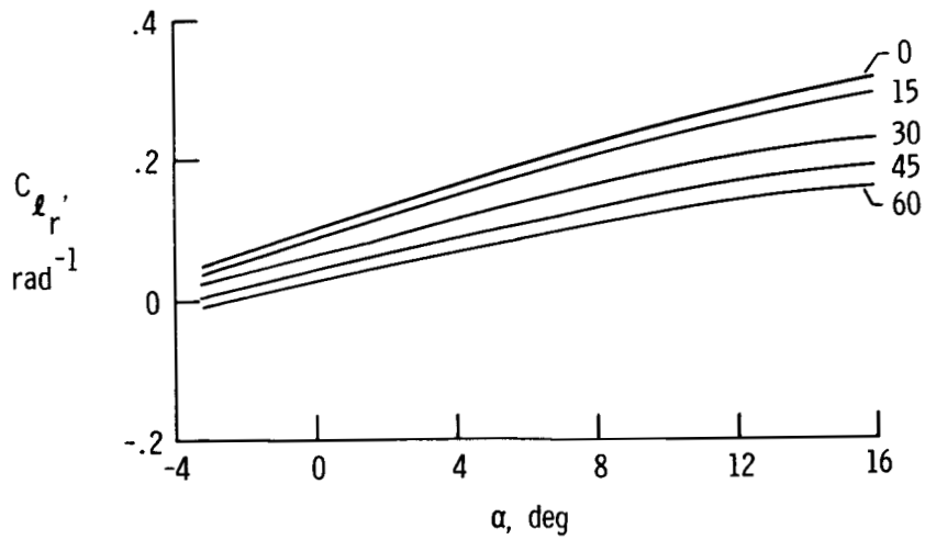
(d) C_{l_q}' , C_{l_p}' , and C_{l_r}' .
