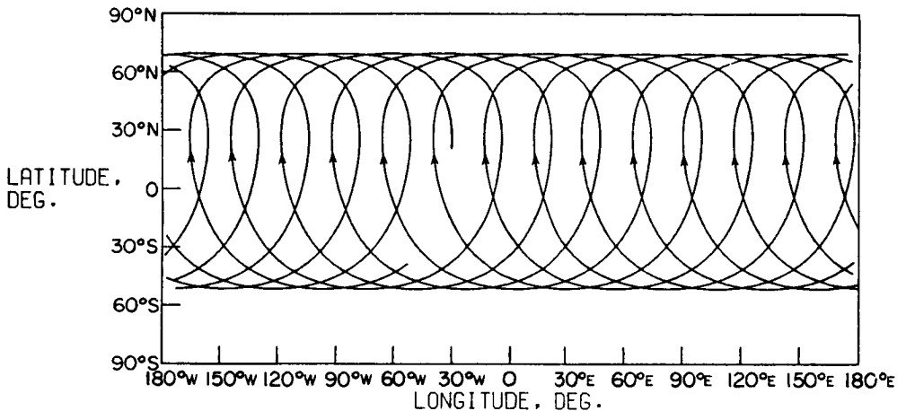
Fig. 3 - Typical SAMS daily latitude versus longitude coverage.
