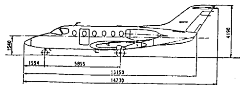
第4図 MU-300 三面図
