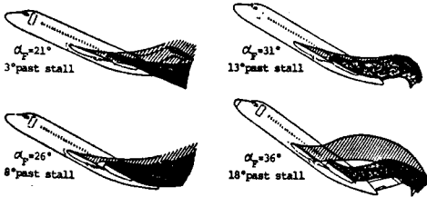
(Fig. 2) ピッチング・モーメント特性と主翼およびナセル後流の関連
