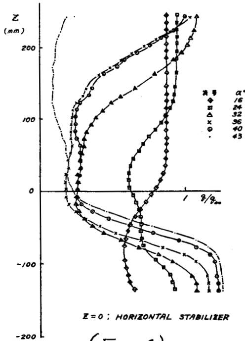
第6図 水平尾翼位置での後流計測結果 (1/12.5 模型寸度)
