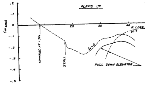
第7図 MU-300の高迎角ピッチング・モーメント特性
