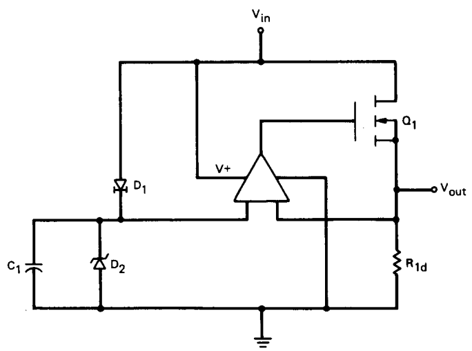
Fig. 2. FET circuit
