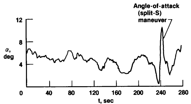
(d) Reference angle of attack.
