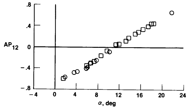
(d) M = 0.90 , orifices on nose cap.
