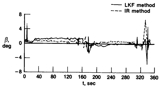
(d) Angle of sideslip.
