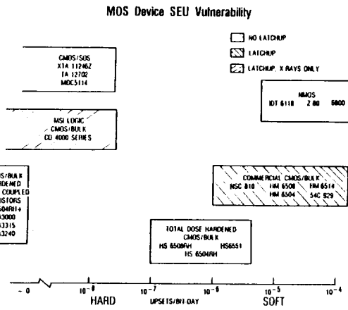
Fig. 15. SEU Rates for MOS Devices
