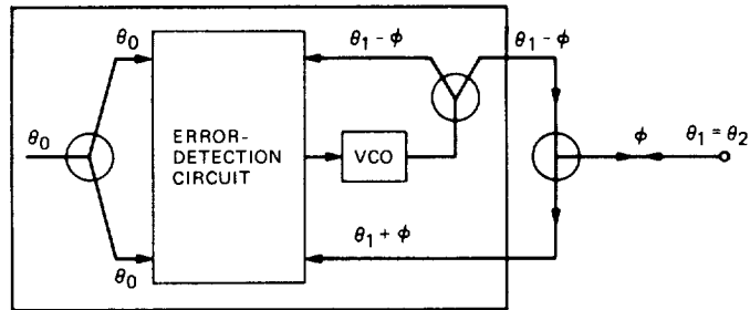
Fig. 2. Phase conjugator.
