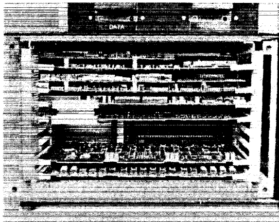
Fig. 13 BSC cardcage.
