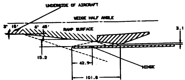
Fig. 8a. Scramjet Inlet M = 6.0
