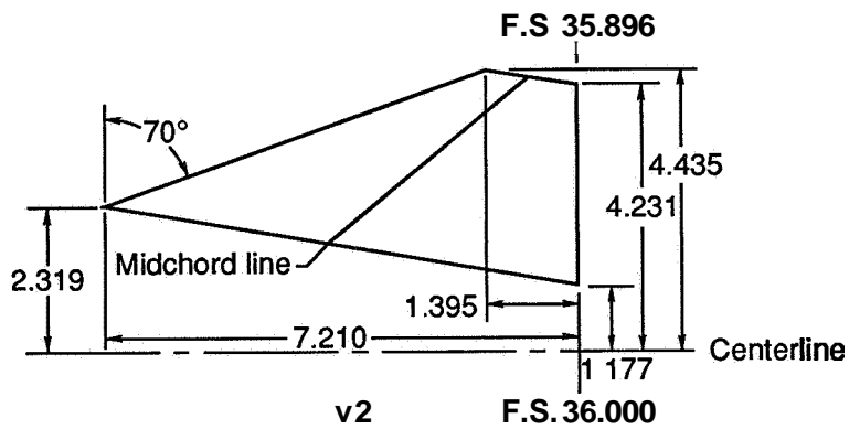
(d) Details of centerline-mounted vertical tails.
