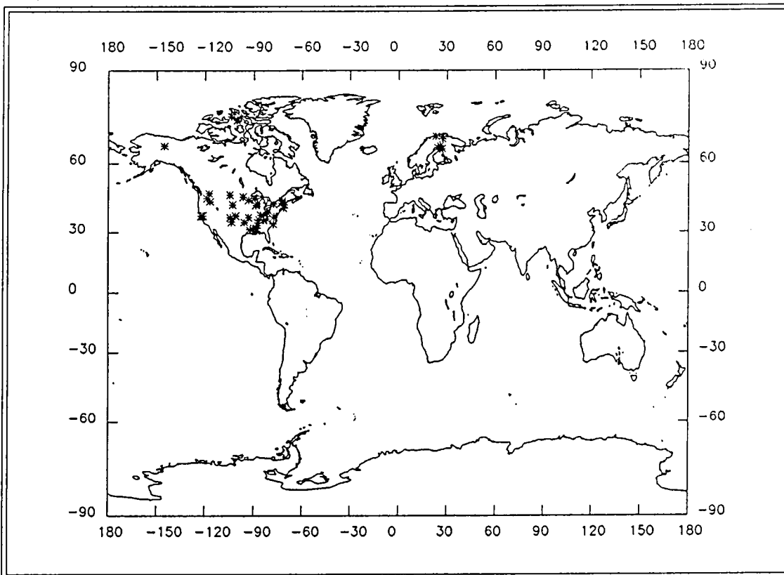
Figure 7 continued... (c) 1912.5 - 1917.5, and (d) 1917.5 - 1922.5
