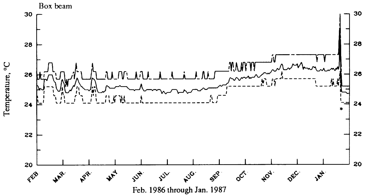
(d) Passive analog temperatures.
