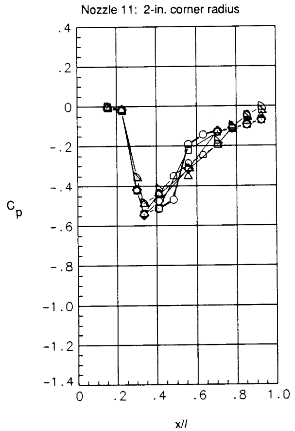
(d) Pressure distributions at M_\infty = 1.2 .
