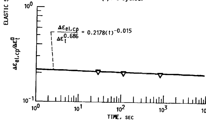
(b) CP cycles.
