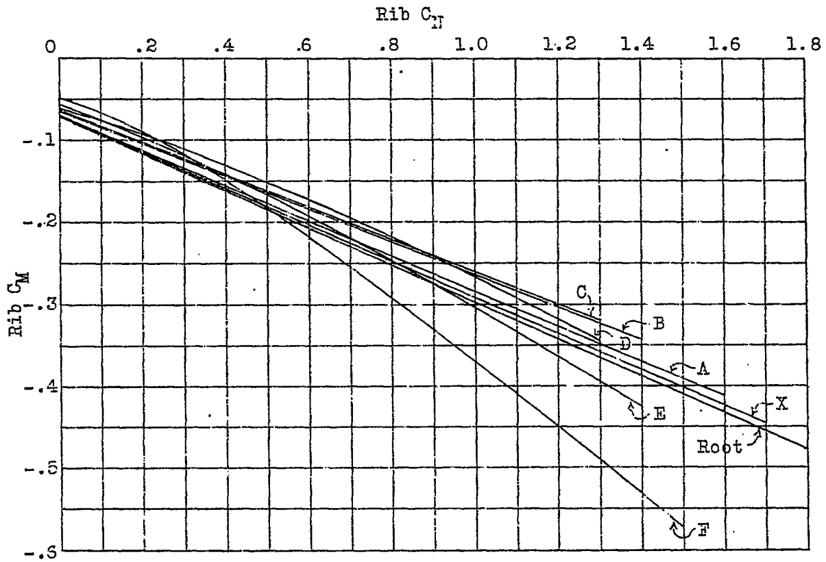
Rib C_M vs. rib C_N
