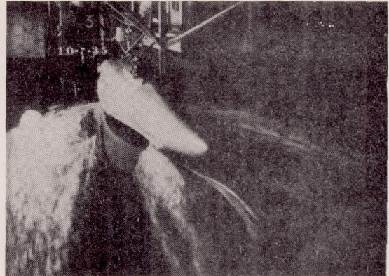
(d) C_{\Delta} = 0.2 ; C_V = 1.95 ; \tau = 9^{\circ}
