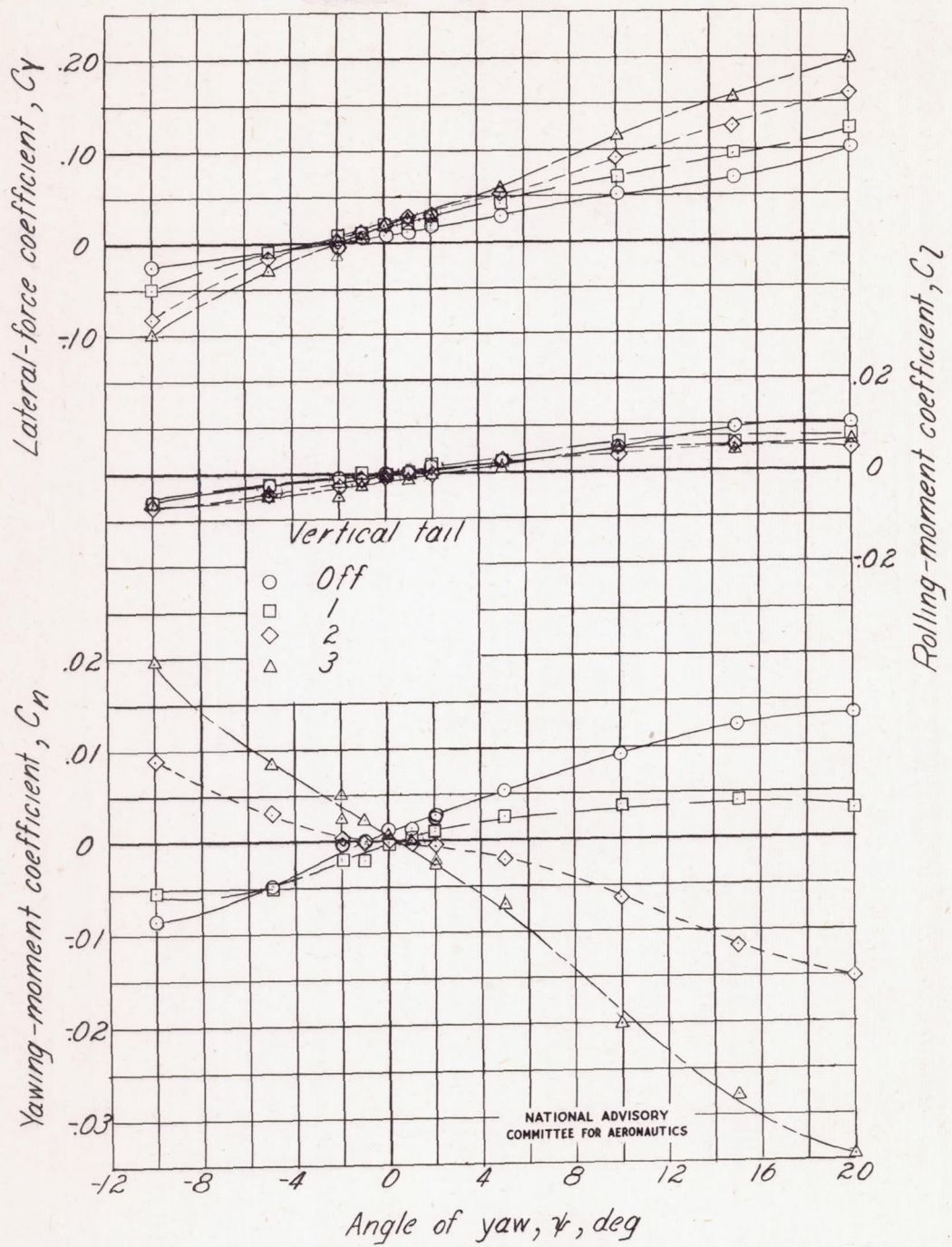
(d) Large box canopy ; \alpha = 10.6^\circ .
