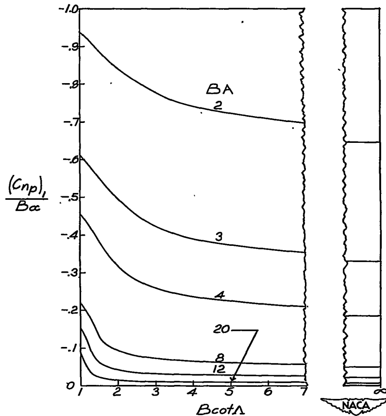
(d) Taper ratio \lambda = 1.0 .
