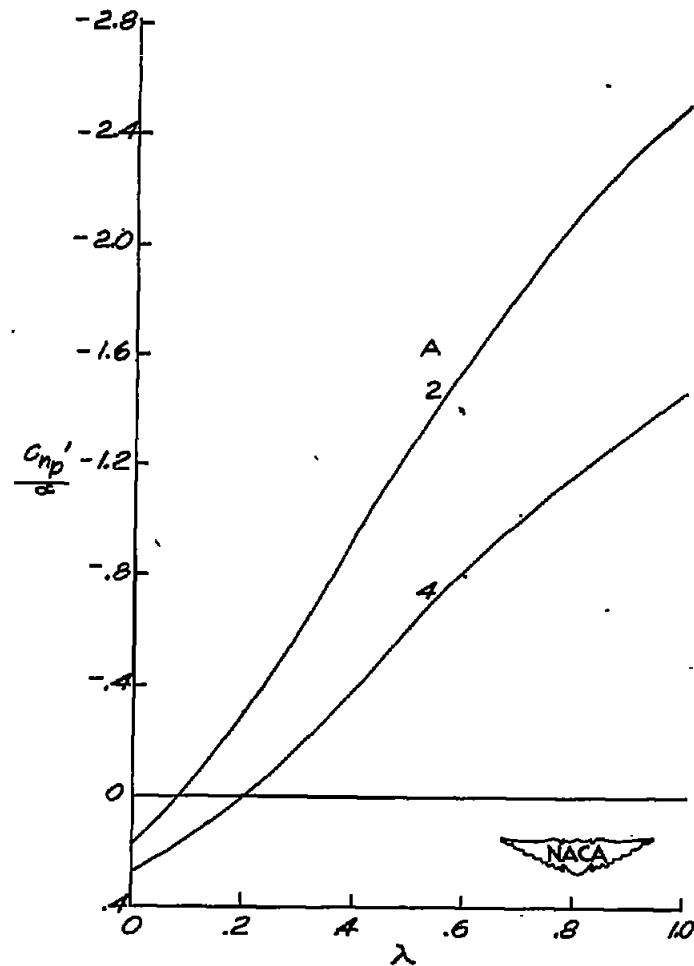
(d) Variation with taper ratio. M = 2; Λ = 53°.
