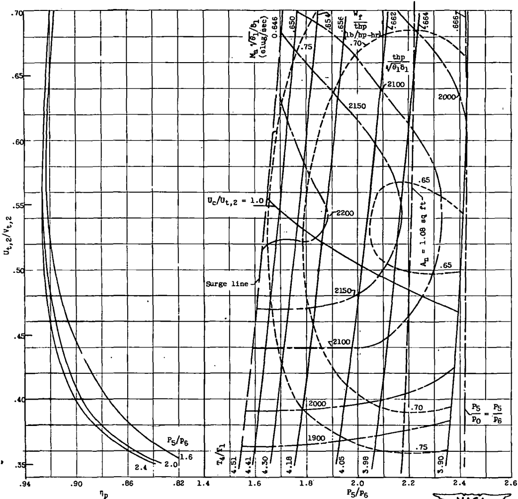
(d) U_c/\sqrt{t_{t,2}} , 1006 feet per second; Y , 0.06 (flight Mach number, 0.55).
