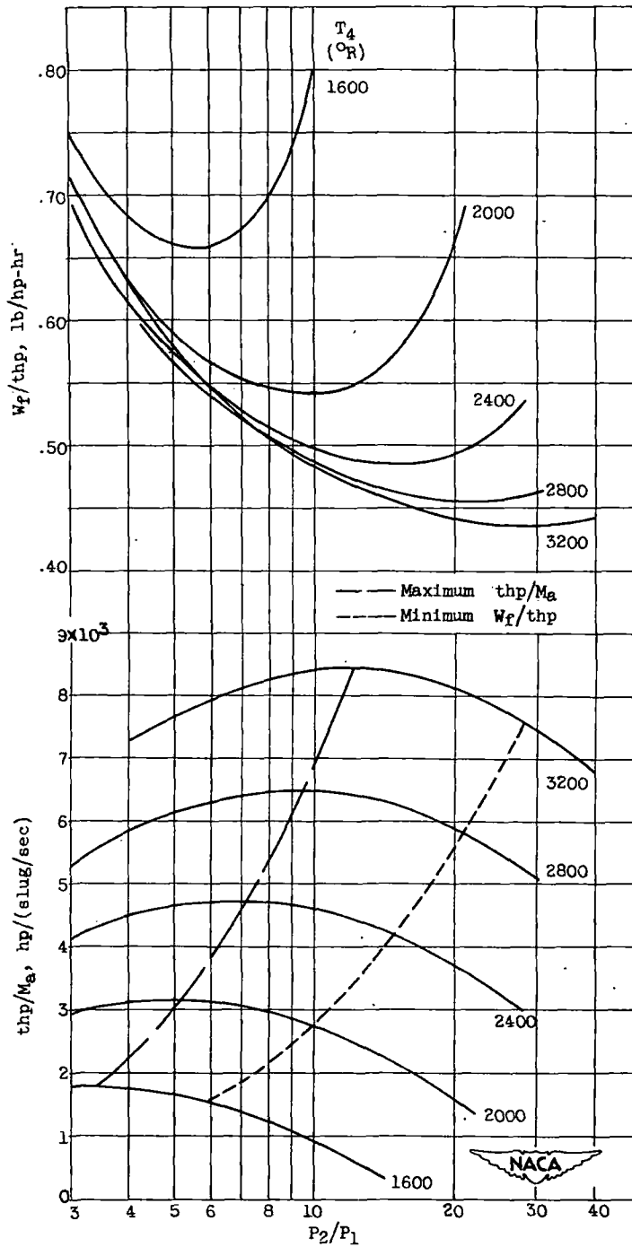
(b) V_0 , 733 feet per second; t_0 , 519° R; V_j , 902 feet per second; \eta_p , 0.85.
