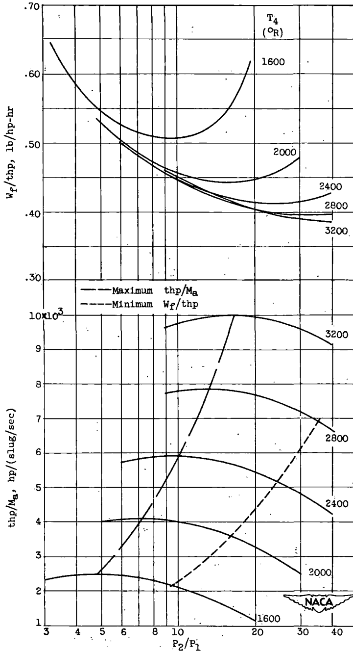
(c) V_0 , 733 feet per second; t_0 , 412° R; V_j , 902 feet per second; \eta_p , 0.85.
