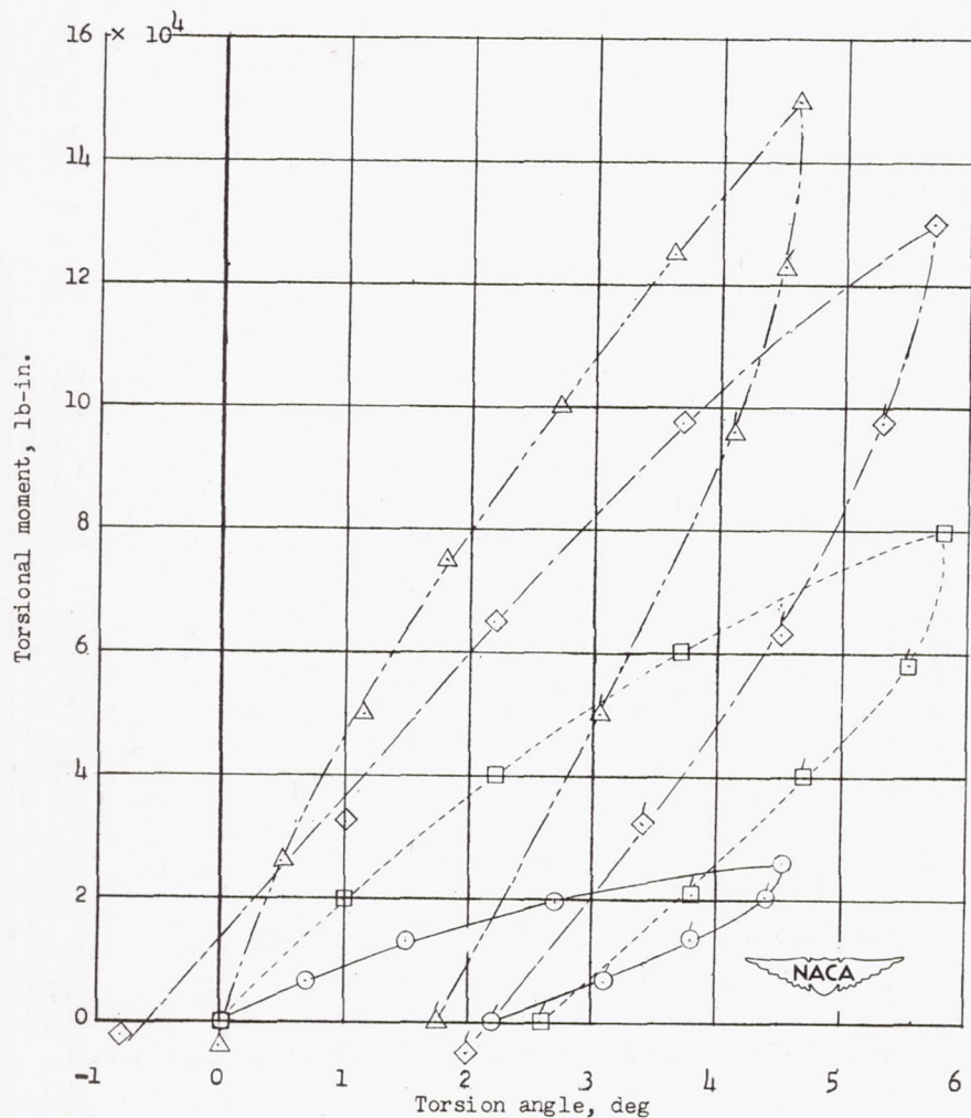
(d) Initial inflation pressure, 180 pounds per square inch.
