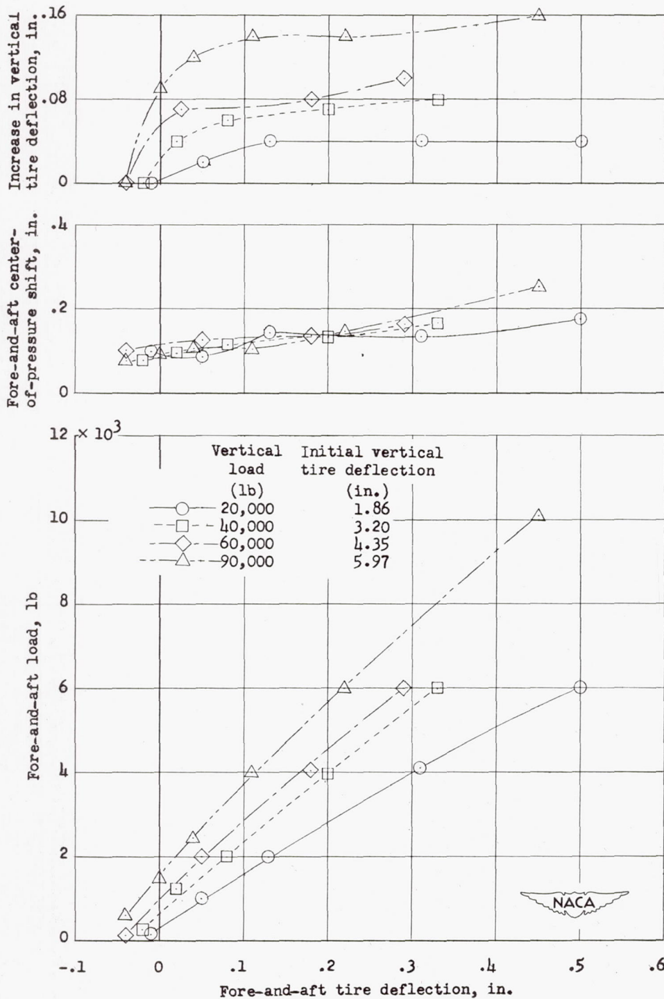
(d) Initial inflation pressure, 180 pounds per square inch.
