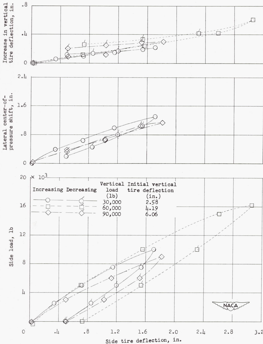
(d) Initial inflation pressure, 180 pounds per square inch.
