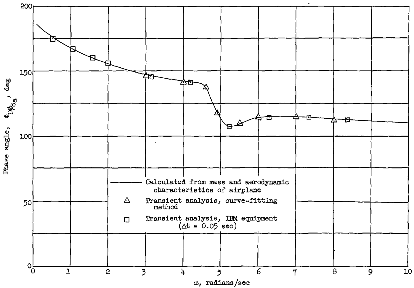
(d) Phase angle \phi_{D\dot{\theta}_a} .
