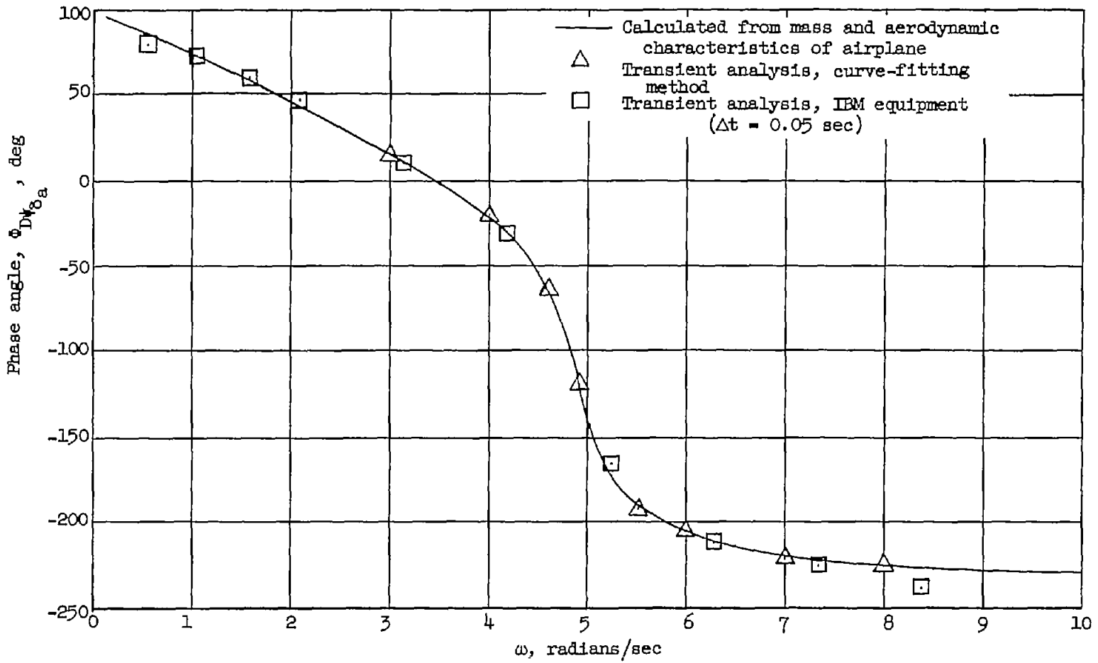
(f) Phase angle \phi_{D\psi_{\delta a}} .
