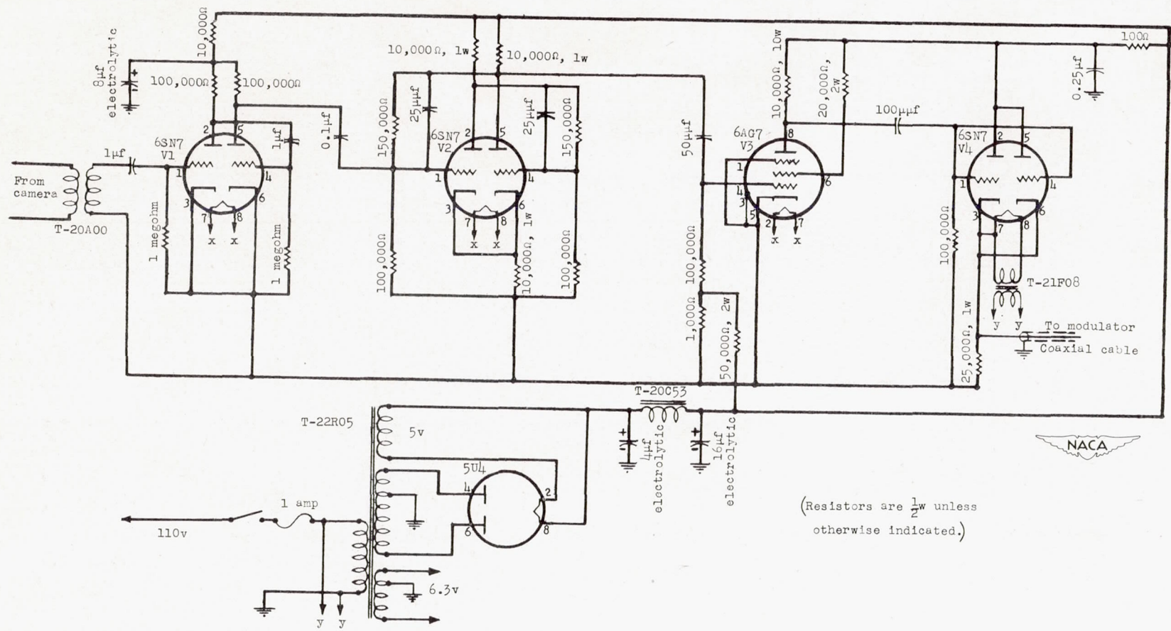
Figure 3.- Pulse amplifier.
