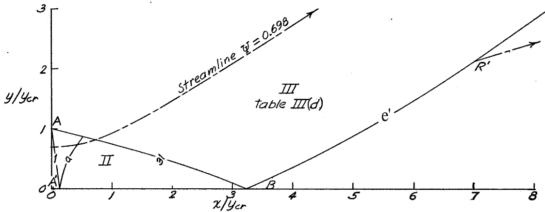
(d) v_B = 40^\circ .
