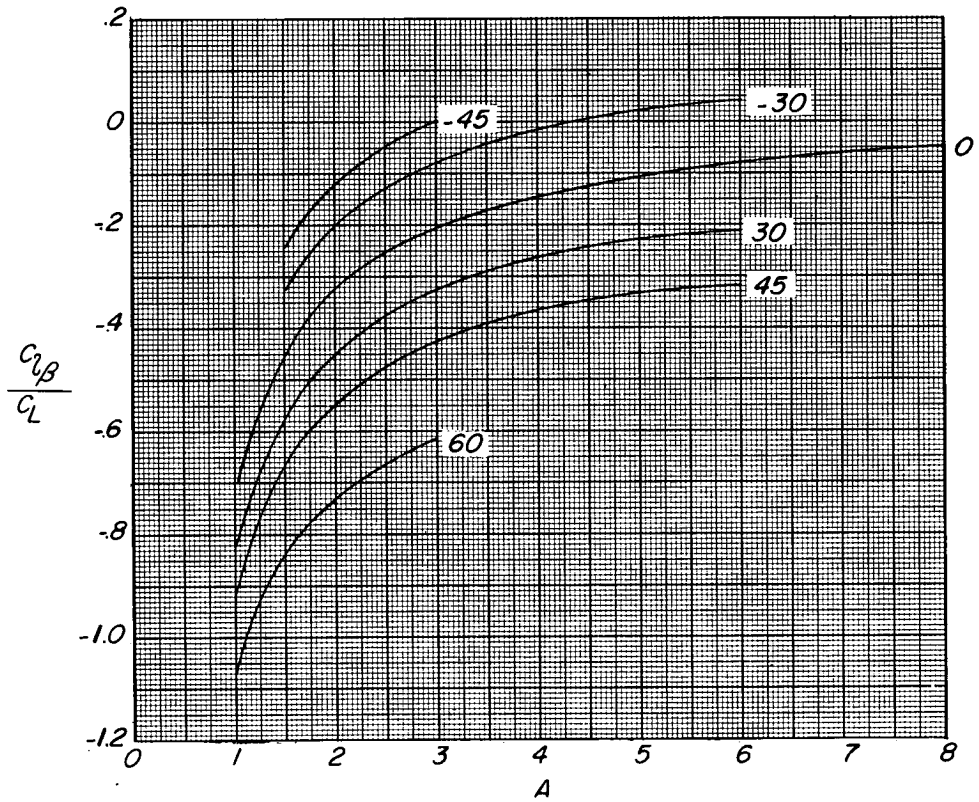
(d) \lambda = 1.00.
