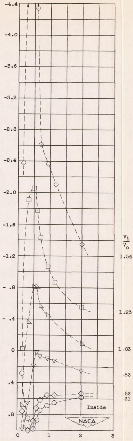
(d) Center-line section - configuration V, C_{Q1} = 1.7 .
