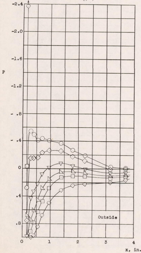
(d) Center-line section - configuration V, C_{Q1} = 1.7 .
