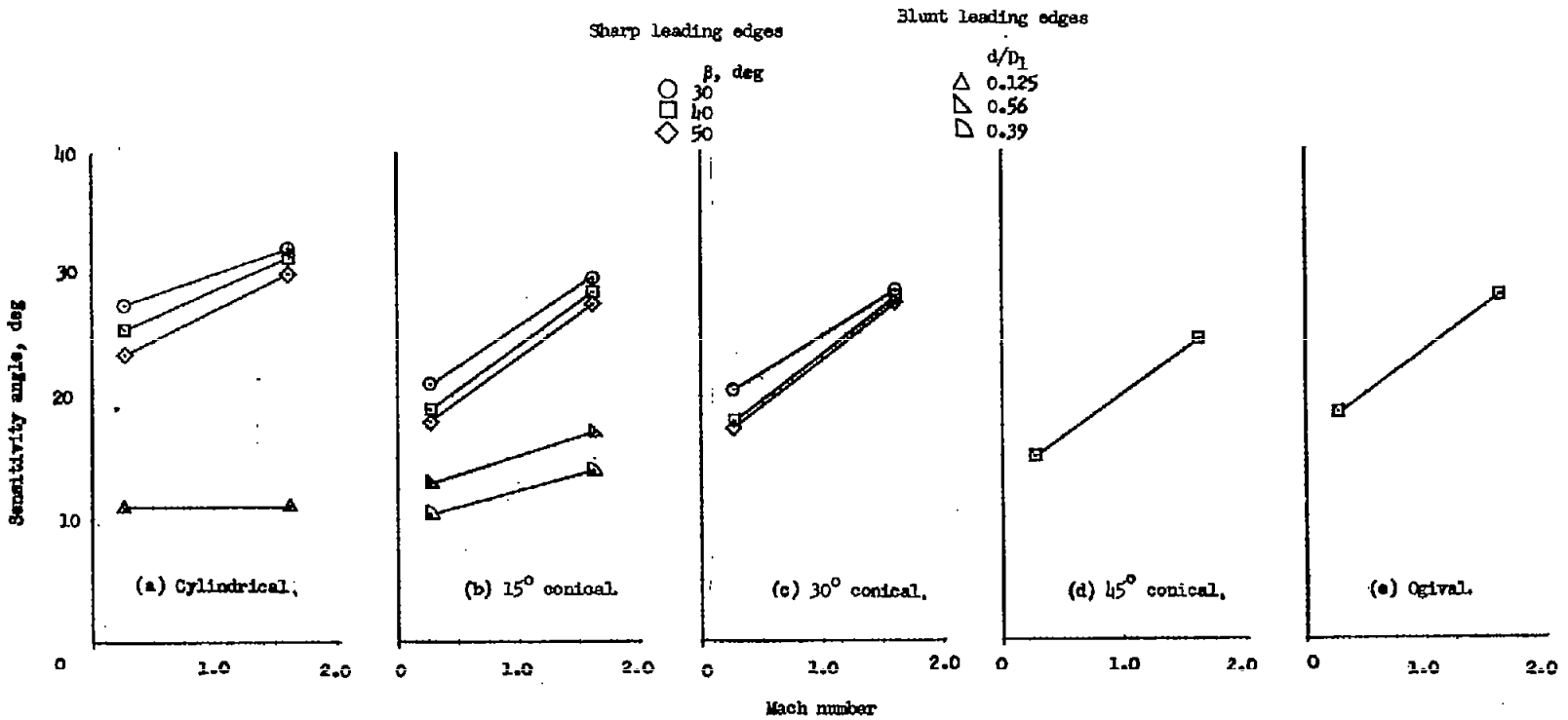
(a) Cylindrical. (b) 15° conical. (c) 30° conical. (d) 45° conical. (e) Ogival.
