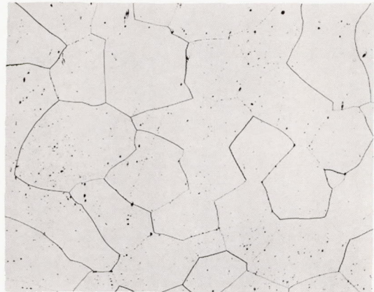
(d) 31.5-Percent-aluminum NiAl, homogenized at 2200° F for 48 hours.
