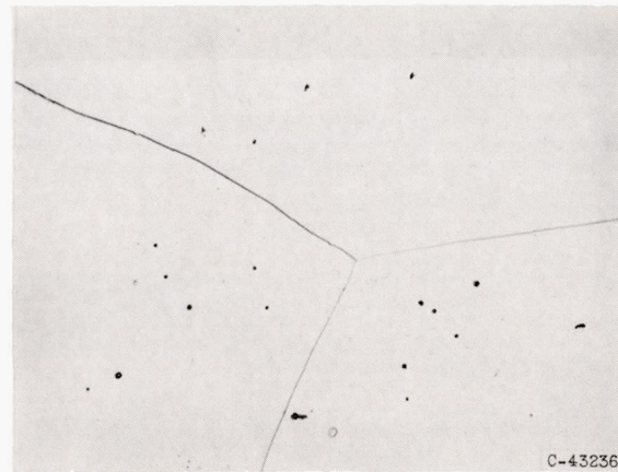
(d) 25-Percent-aluminum NiAl, homogenized at 2400° F for 6 hours.
