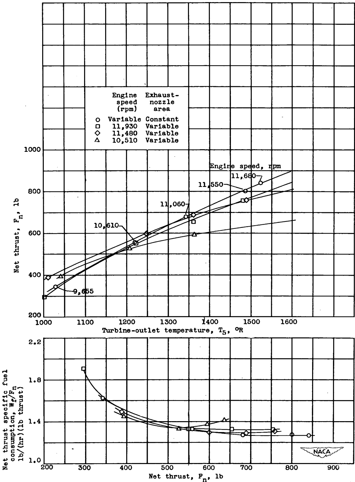
(d) Altitude, 35,000 feet; flight Mach number, 0.52.
