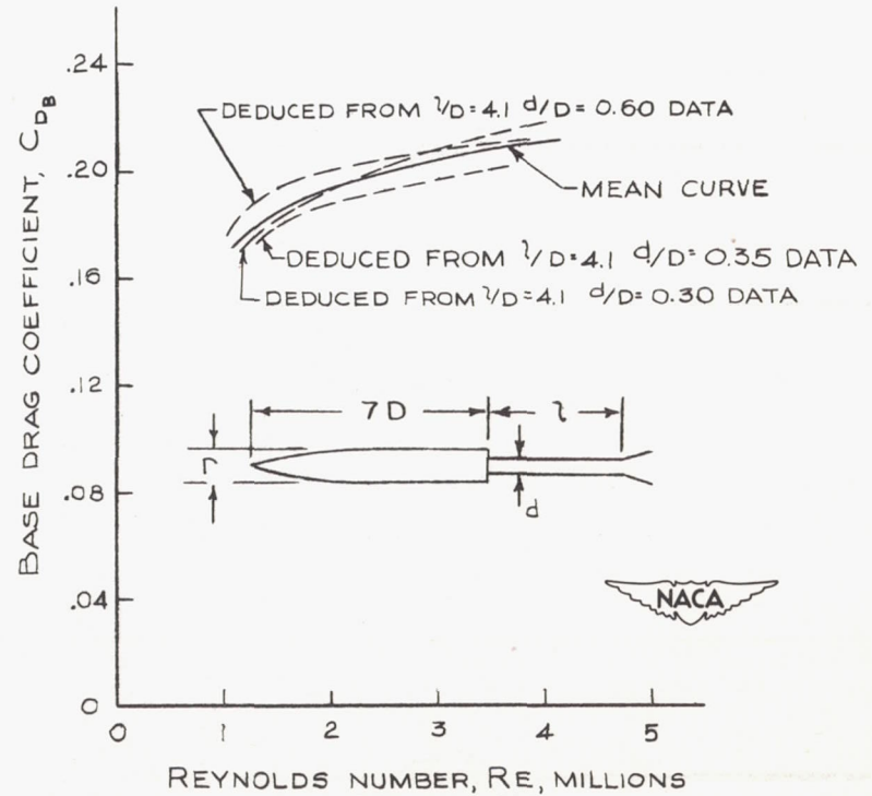
(d) MEAN INTERFERENCE-FREE CURVE.
