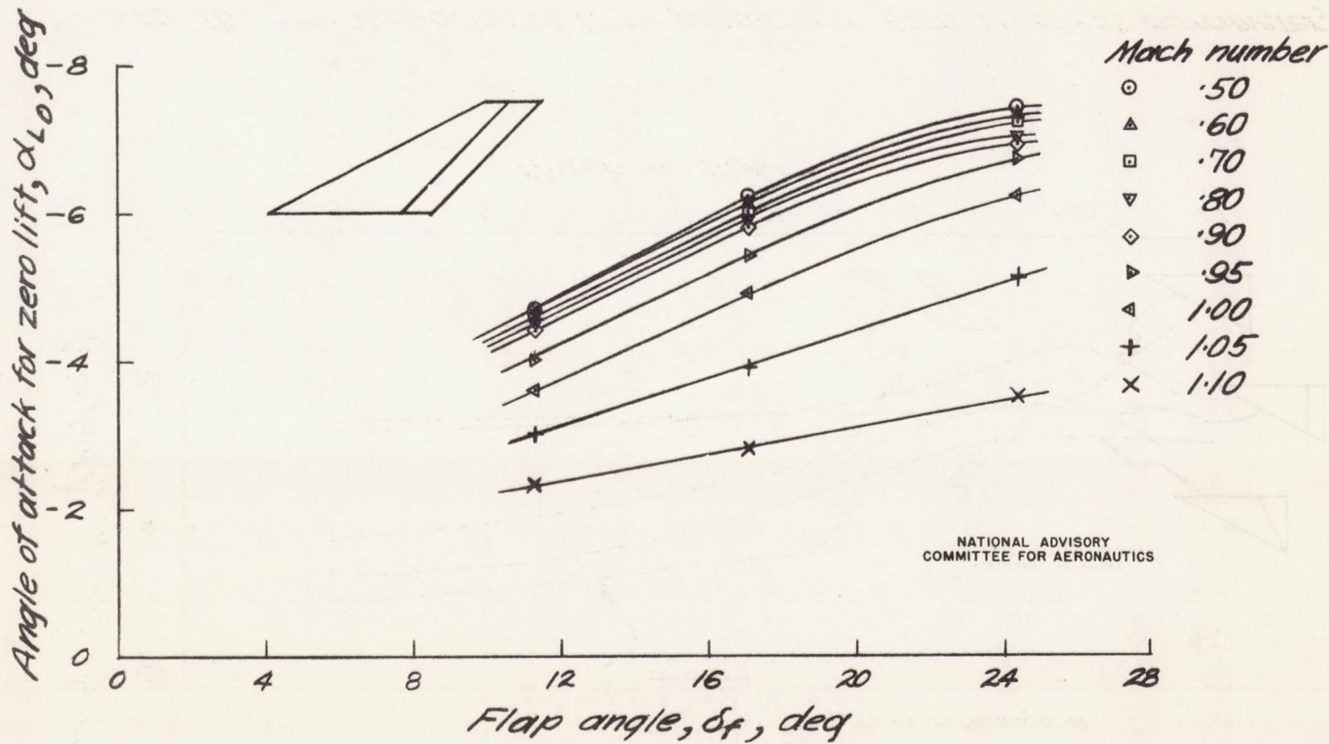
(d) Swept-back constant-chord flap
