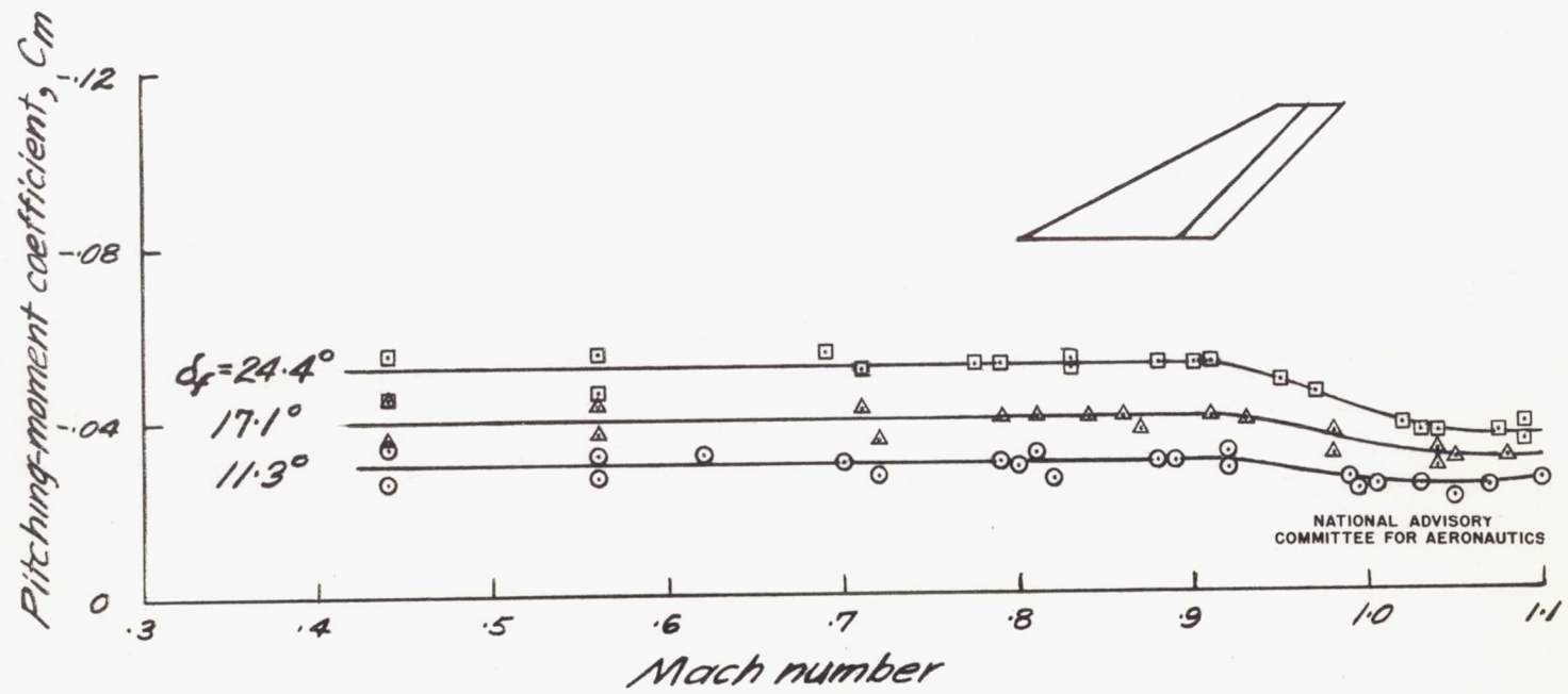
(d) Swept-back constant-chord flap
