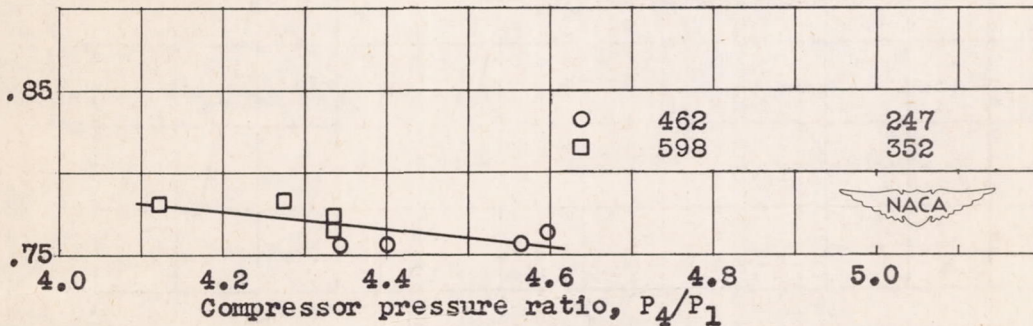
(d) Average compressor-inlet Reynolds number, 68,800.
