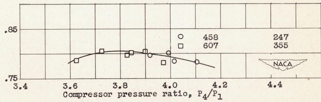
(d) Average compressor-inlet Reynolds number, 65,200.
