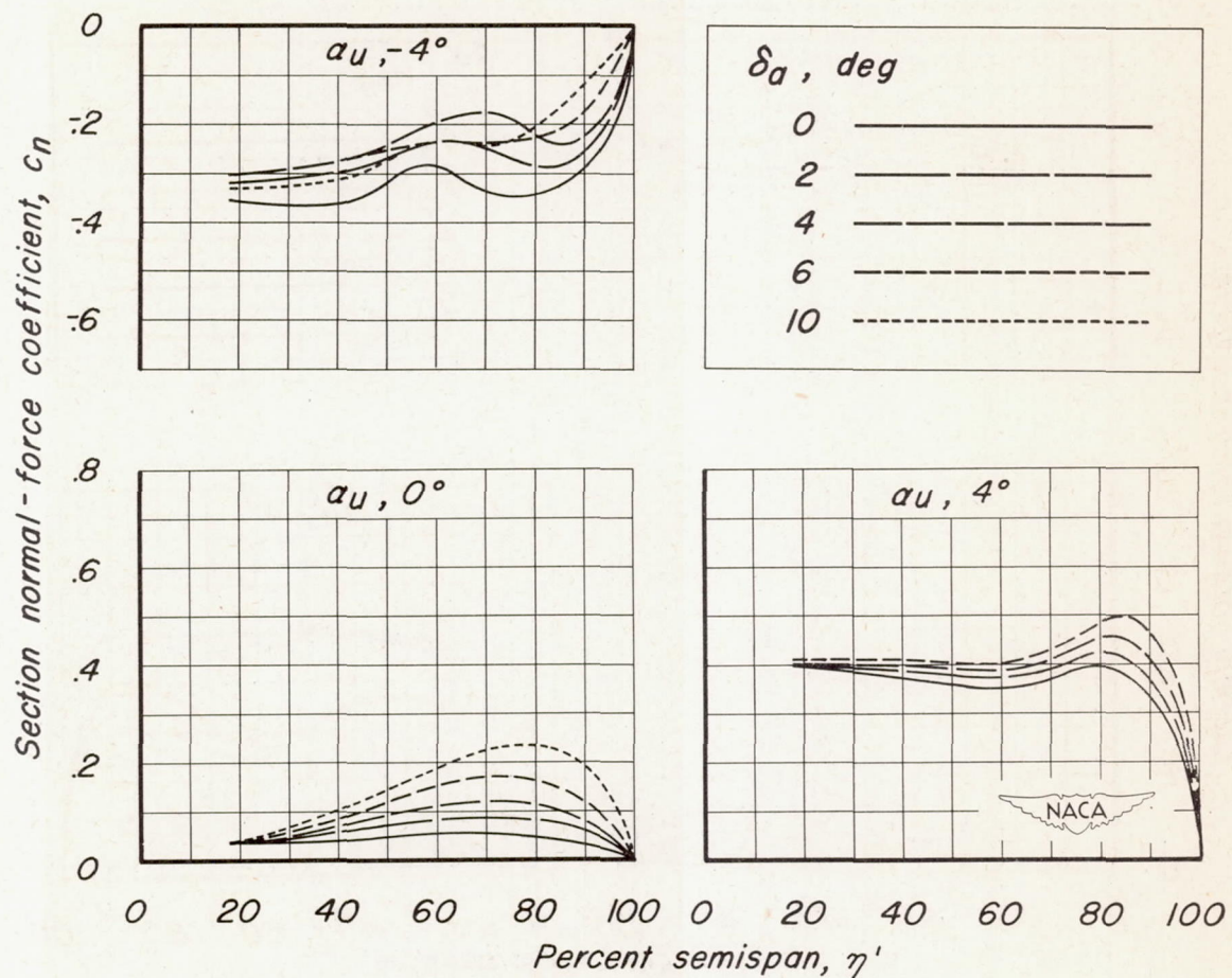
(d) M, 0.85 . Figure 5-Continued.
