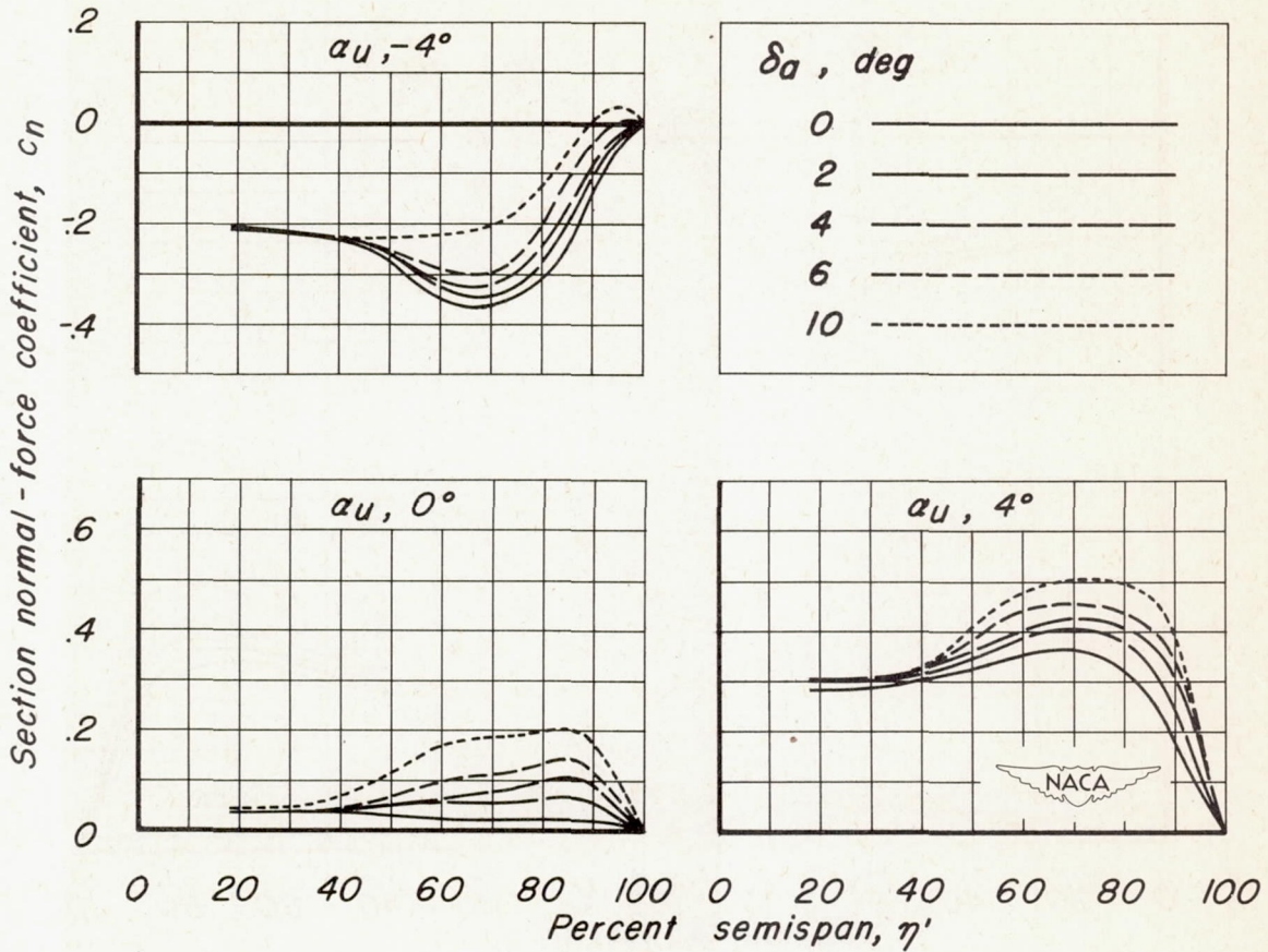
(d) M, 0.85 . Figure 6.-Continued.
