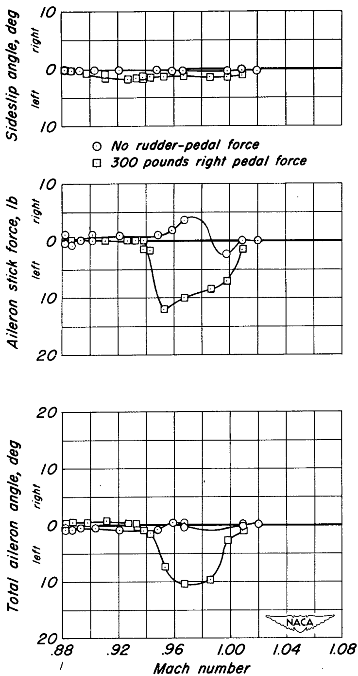
(b) Vortex-generator configuration A.
