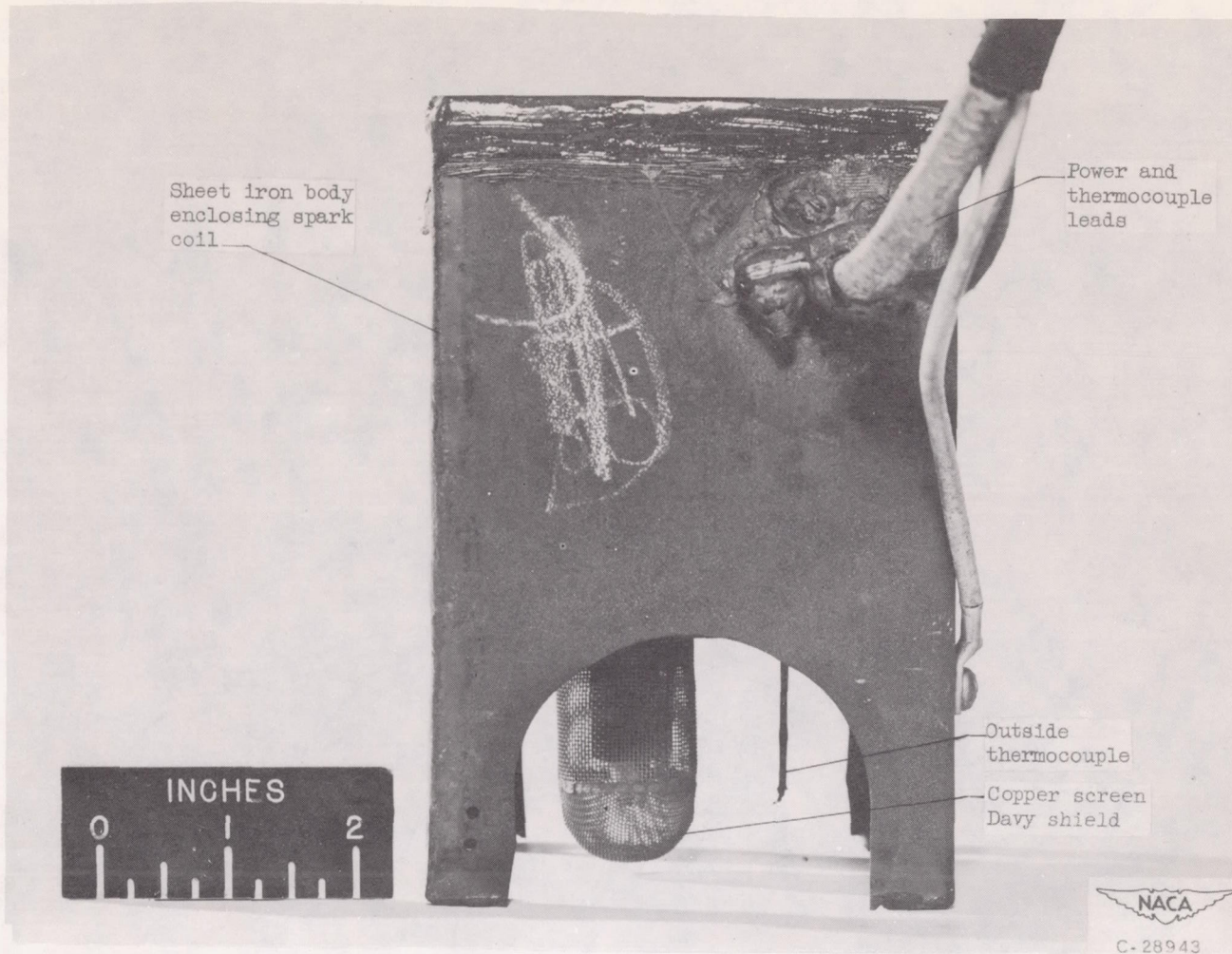
Figure 33. - Vapor Detector.
