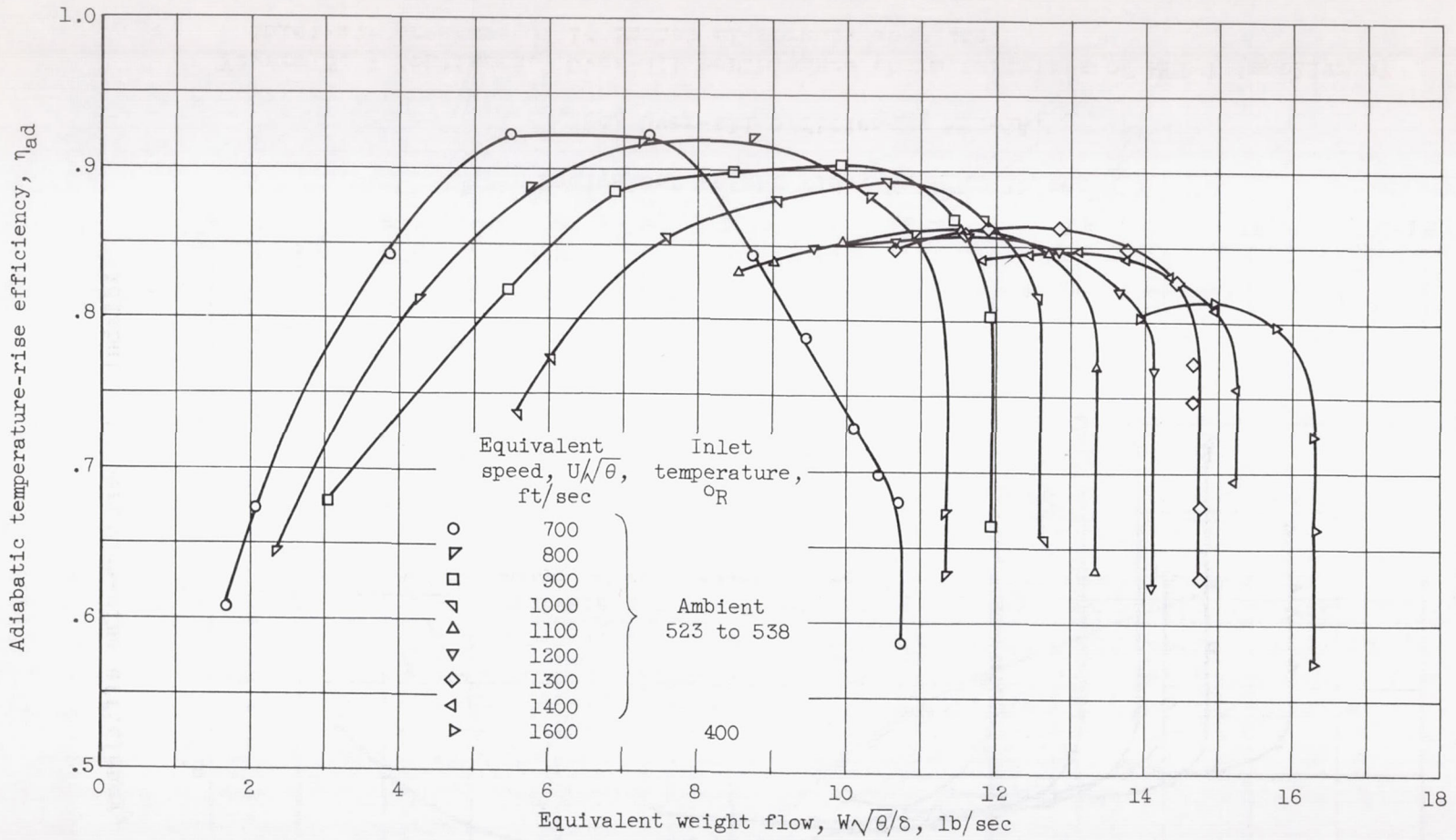
(d) Over-all efficiency, MFI-1B.
