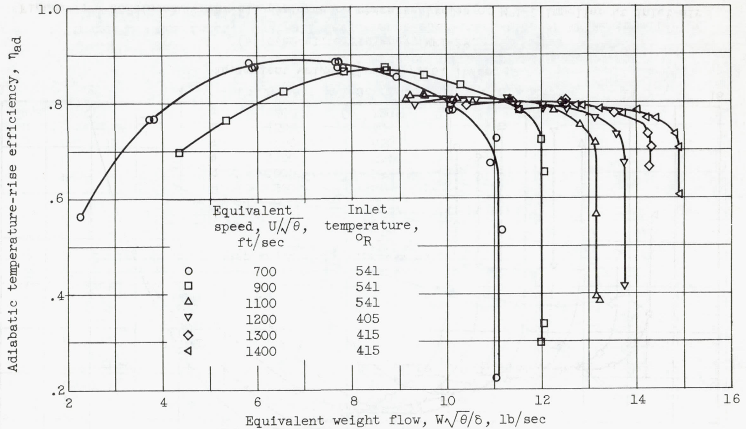
(d) Over-all efficiency, MFI-2A.
