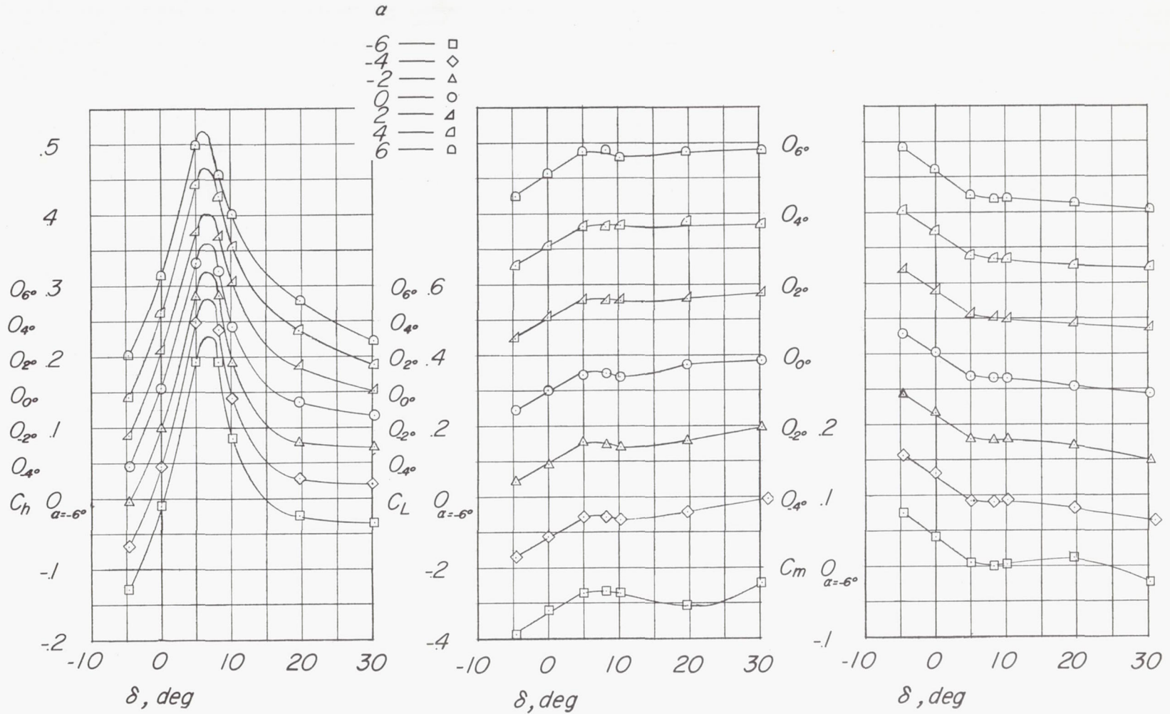
(d) M = 0.85 ; c_b/c_f = 0.79 .
