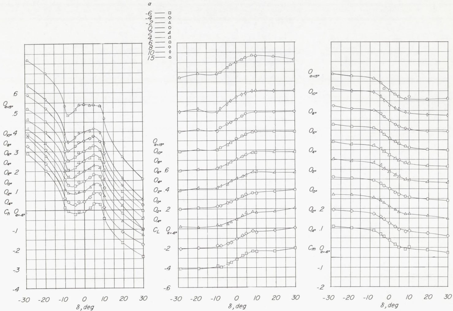
(d) M = 0.85 ; c_b/c_f = 0.50 .
