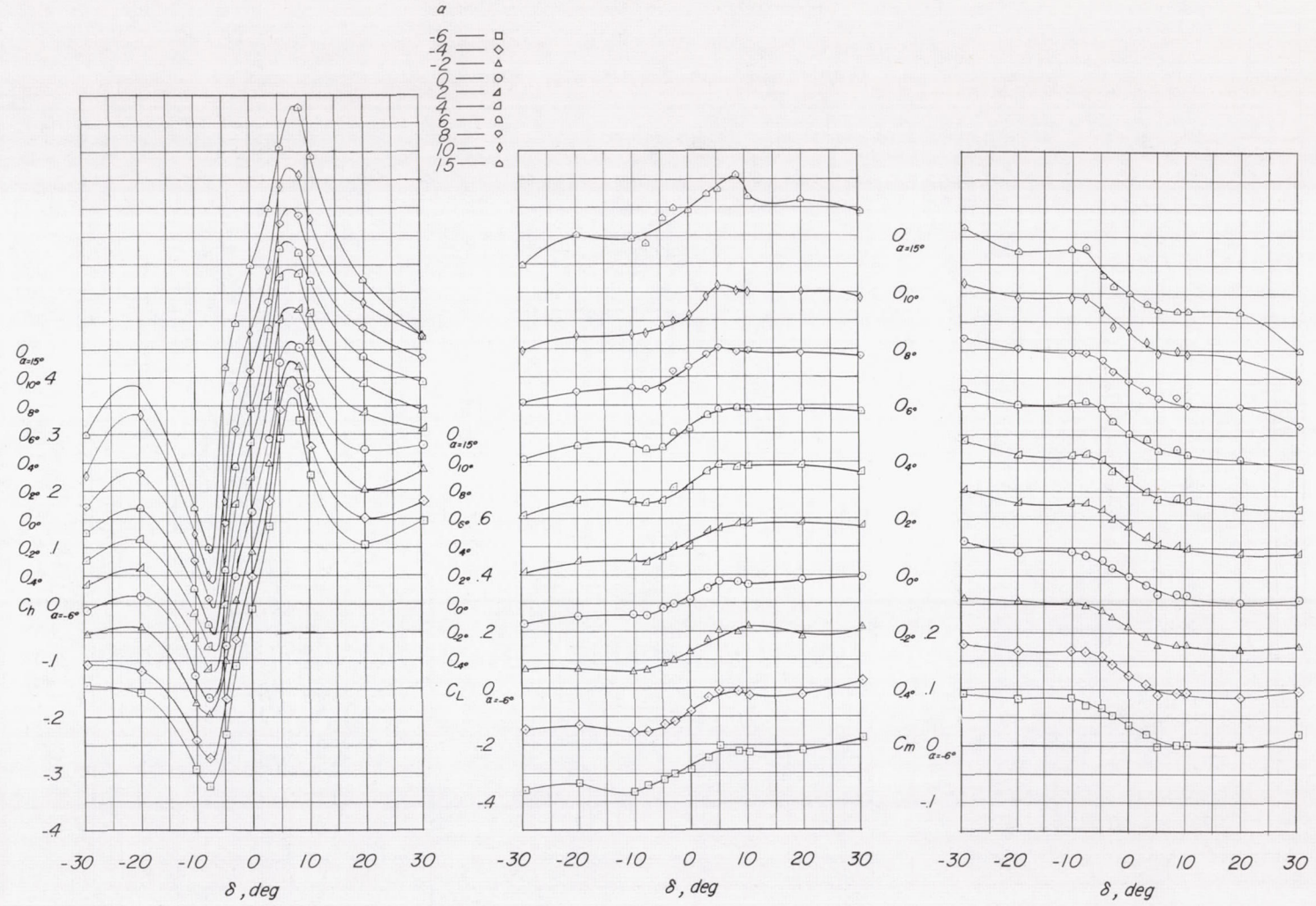
(d) M = 0.85; c_b/c_f = 1.03.
