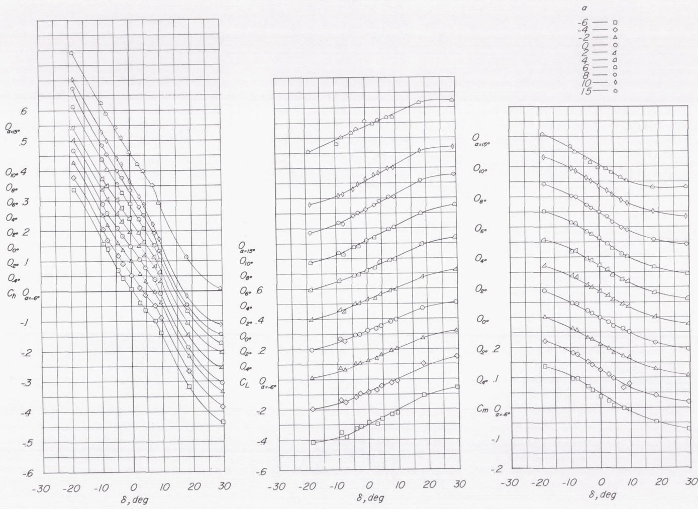
(d) M = 0.85 ; c_b/c_F = 0.07 .
