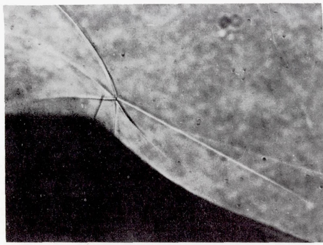
Schlieren
