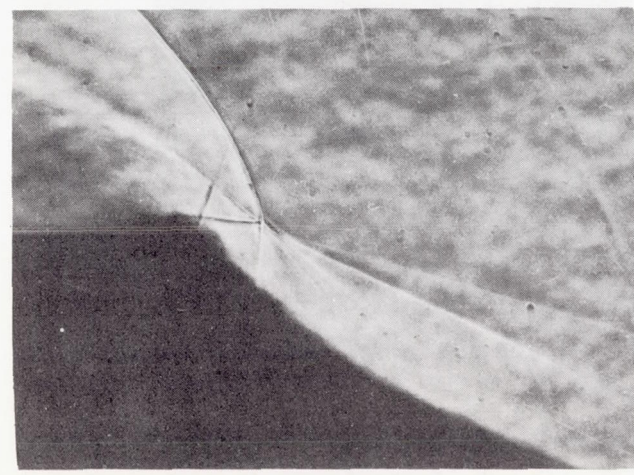
Schlieren
