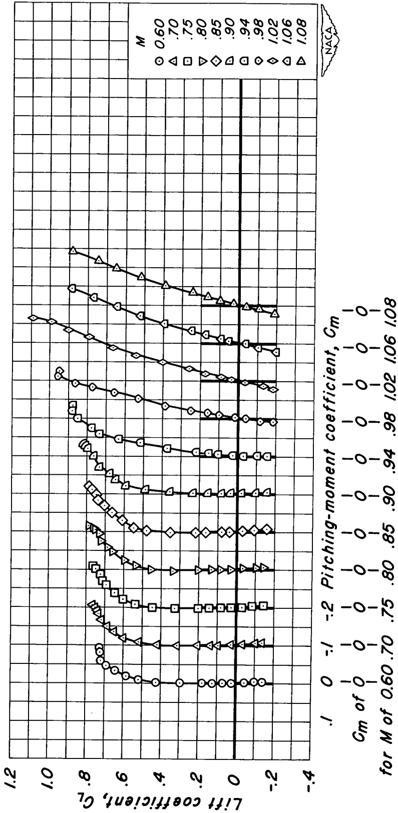
(d) t/c = 0.06 ; \lambda = 0.14
