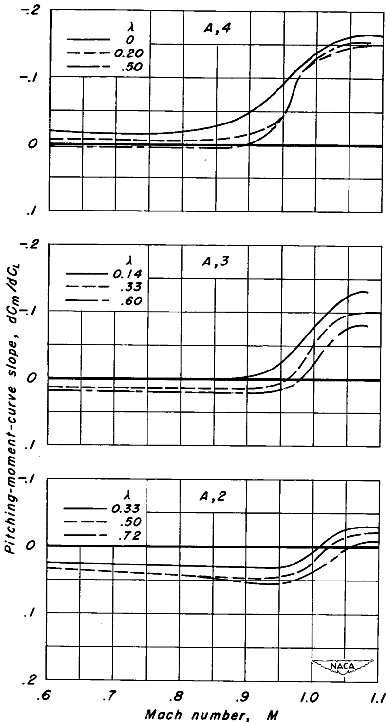
(d) NACA 63A002 sections.
