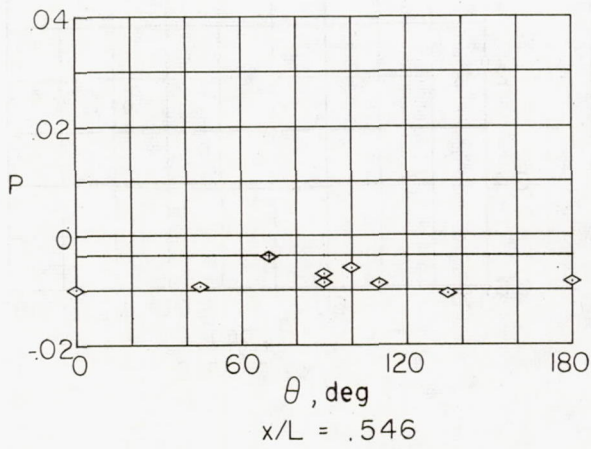
(b) Elliptical body (major axis horizontal).
