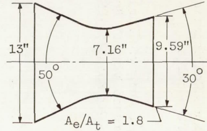
(d) 30° Nozzle.
