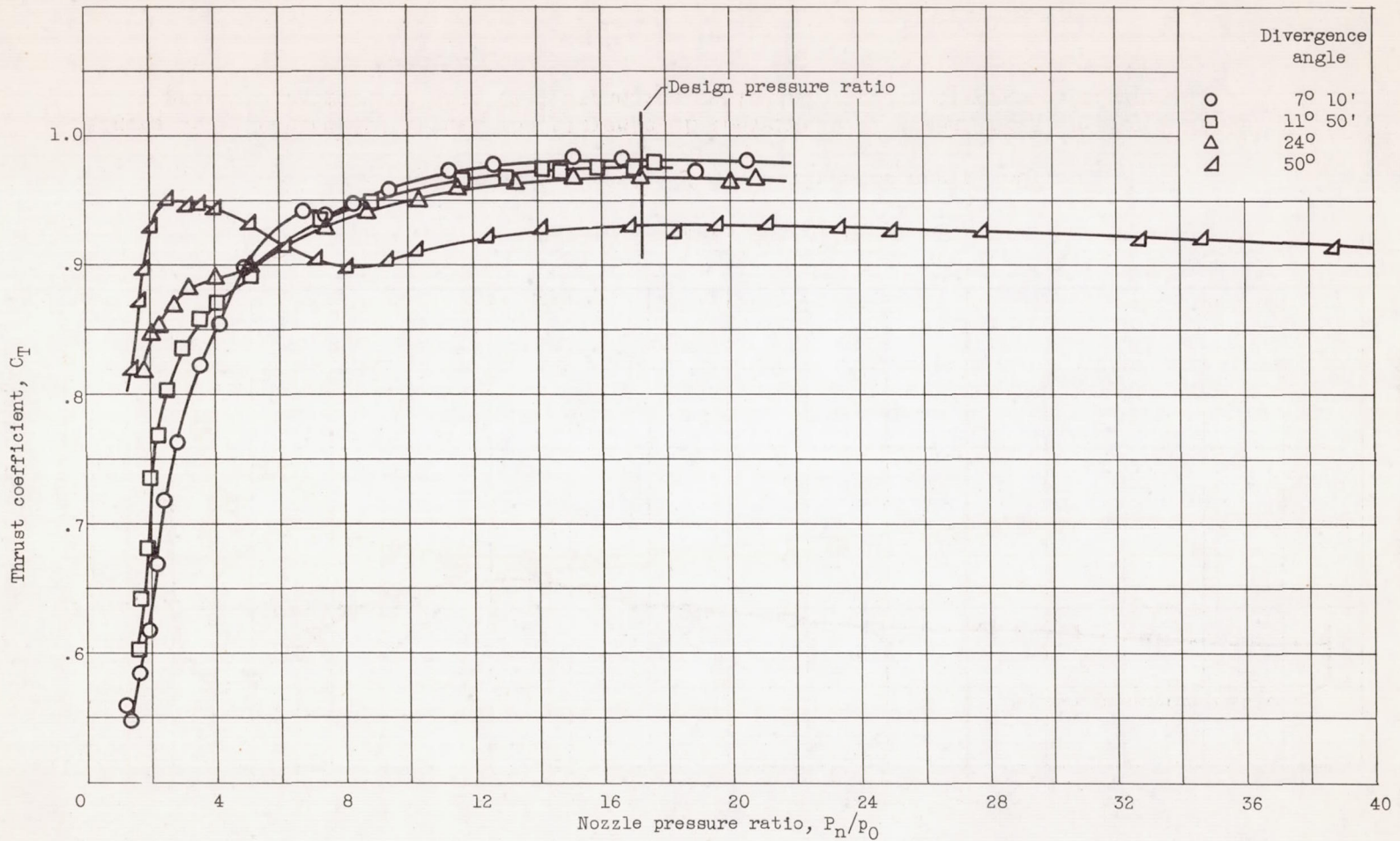
(d) Expansion ratio, 2.65; divergence angles, 7^\circ 10' , 11^\circ 50' , 24^\circ , and 50^\circ .
