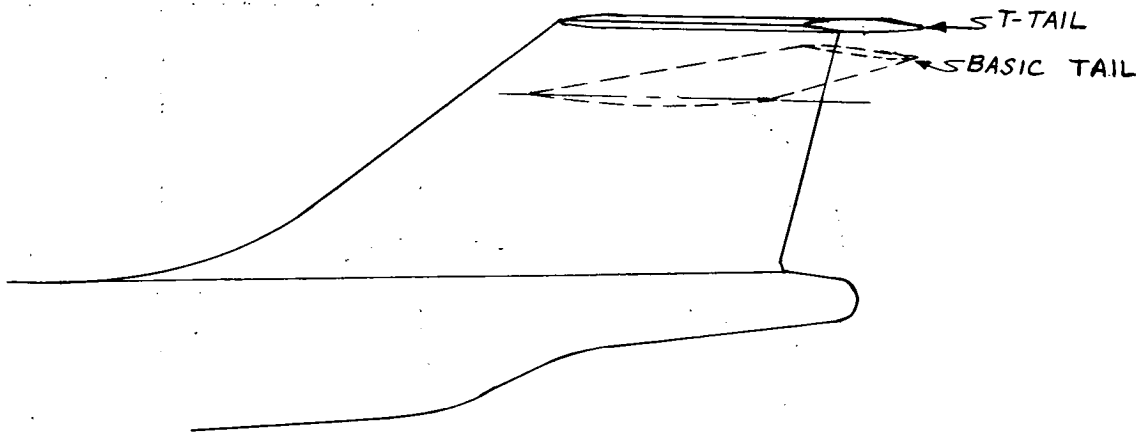
(d) T-tail.
