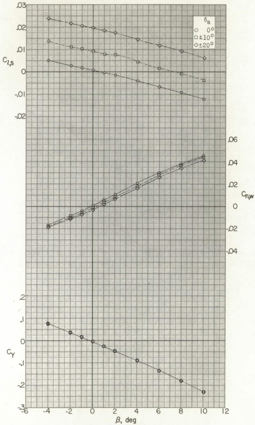
(b) M = 1.56; \alpha = 9.7^\circ .
