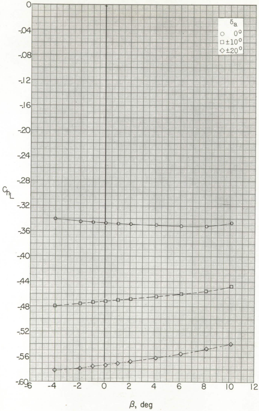
(d) M = 1.56; \alpha \approx 16.2^\circ .
