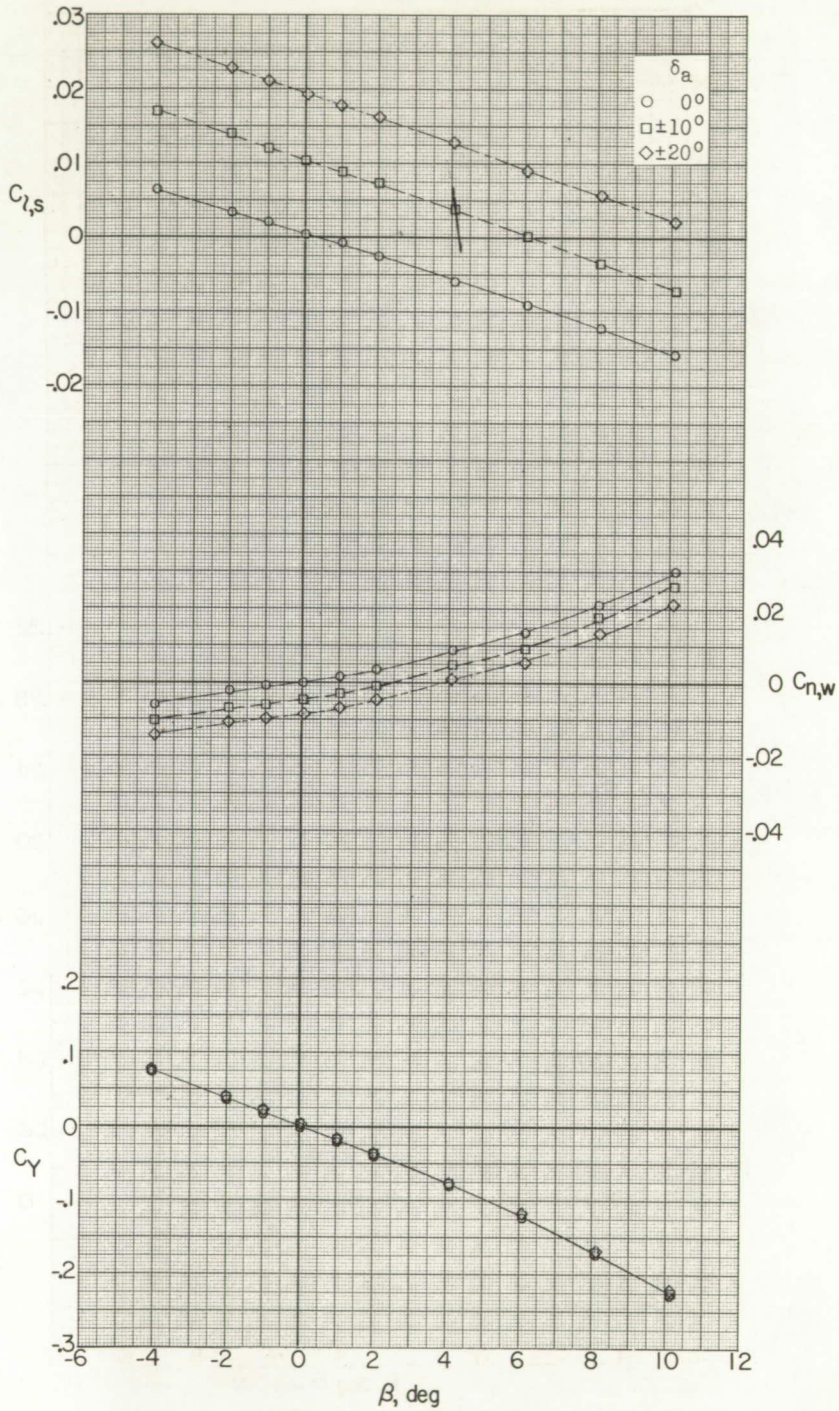
(d) M = 1.56; \alpha \approx 16.2^\circ .
