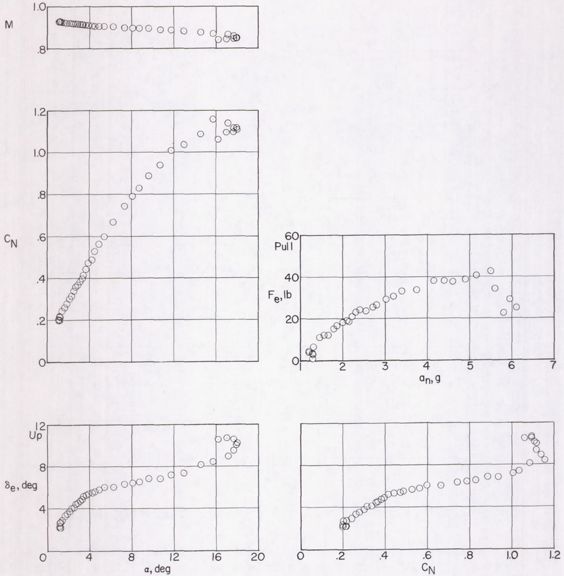
(d) h_p \approx 27,000 feet; i_t = 1.3^\circ ; center of gravity at 0.265\bar{c} .
