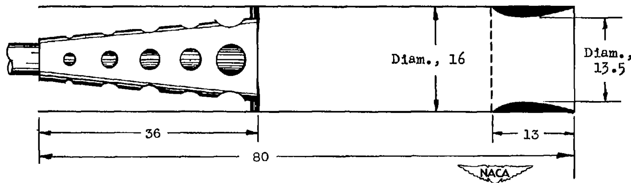
Combustor E
