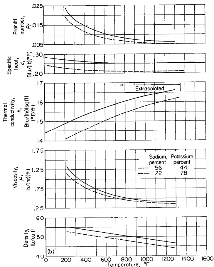
(b) Sodium-potassium alloy.
