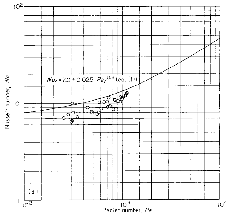
(d) Test section D (length-diameter ratio l/D , 159).
