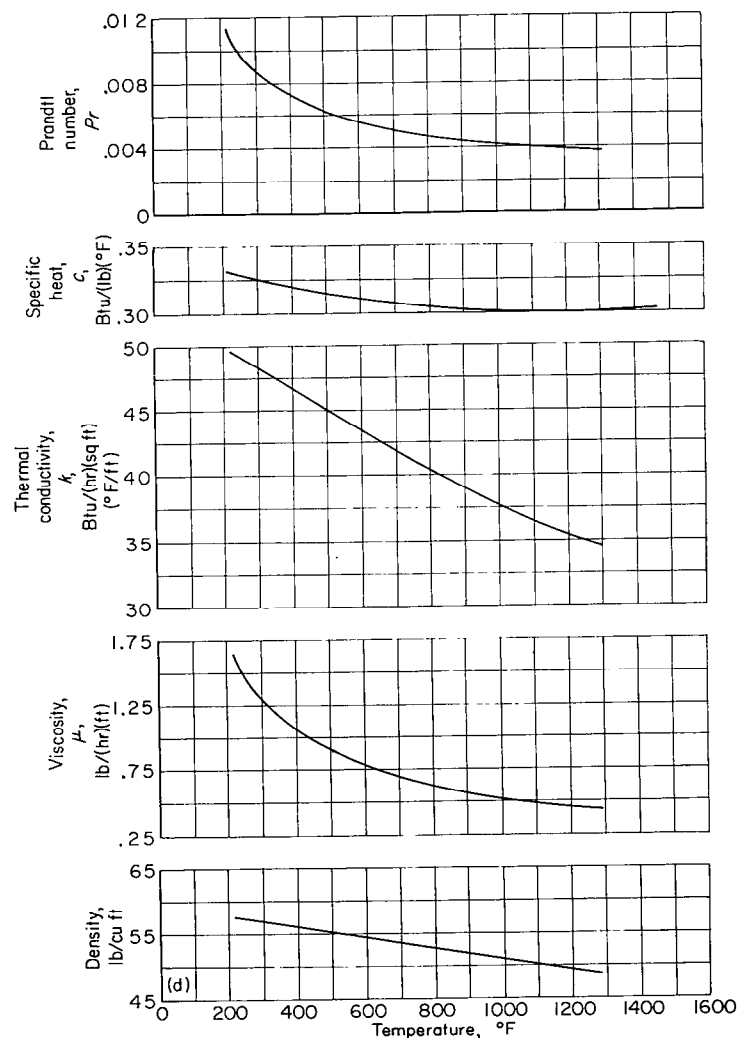
(d) Sodium.
