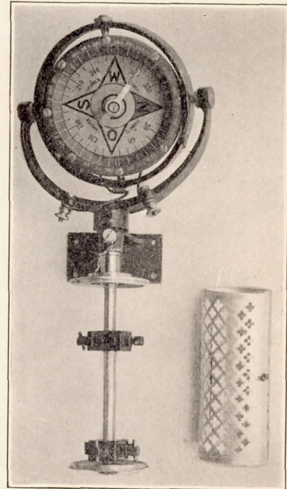
FIG. 21.—Sendtner Armeekompass III.
