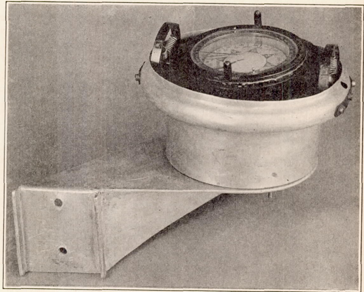
FIG. 24.—Pfadfinder kompass für aviatik.
