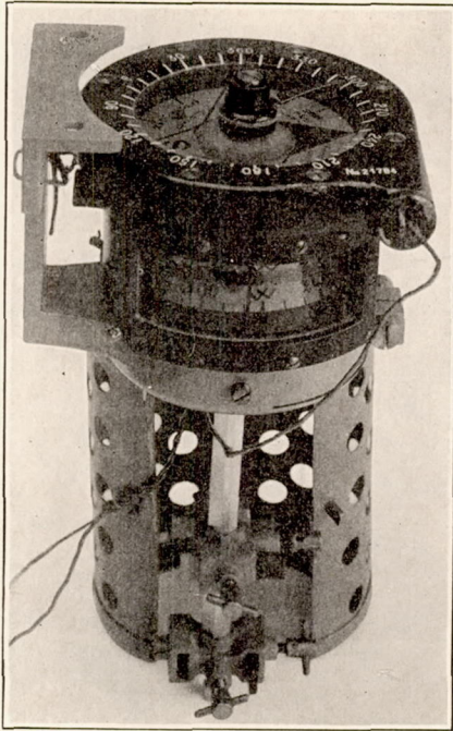
FIG. 23.—Pfadfinder armee kompass IV.
