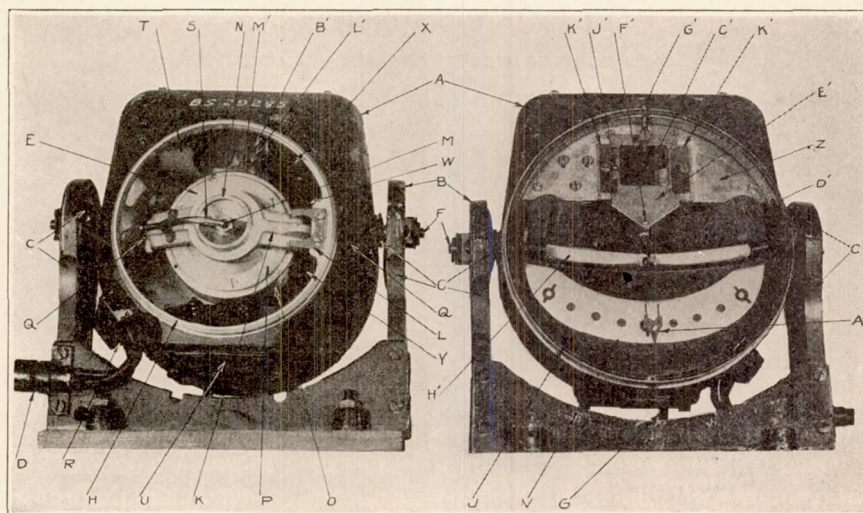
FIG. 18.—Drexler steering gauge.
