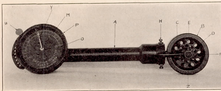
FIG. 13.—R. A. E. turn indicator. Mark V.
