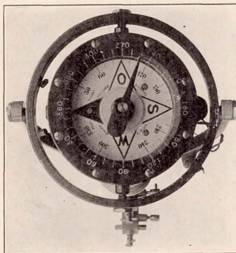
FIG. 22.—Pfadfinder armee kompass III.
