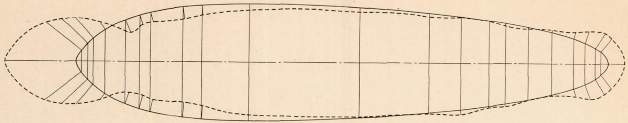
Longitudinal section at E
