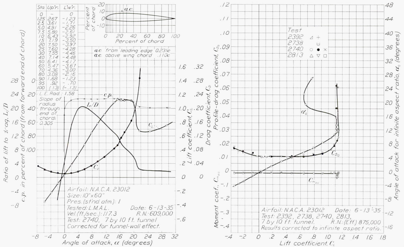
FIGURE 13.—The N. A. C. A. 23012 airfoil.
