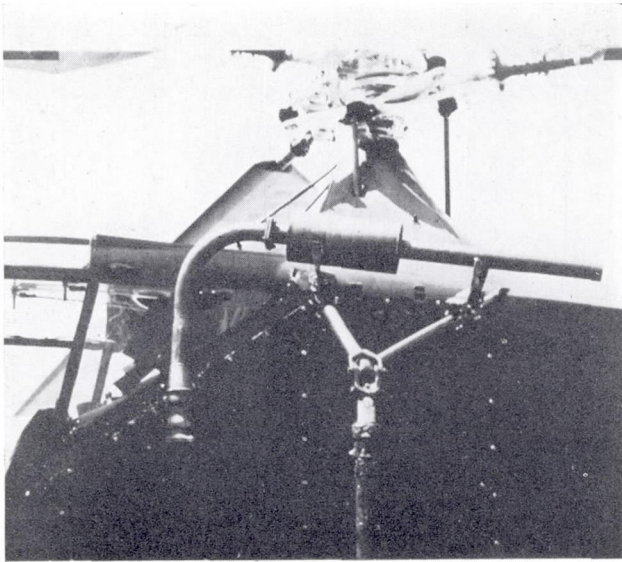
Muffler 78
