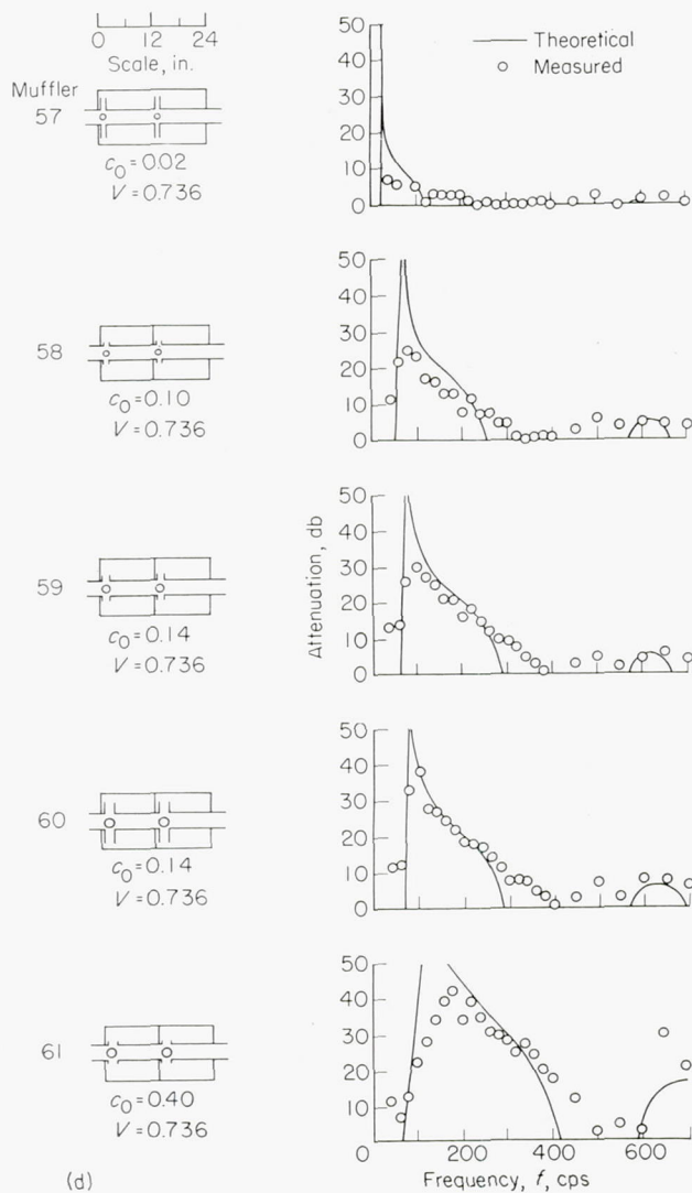
(d) Effect of conductivity c_0 using tubes. Equation (B15).
