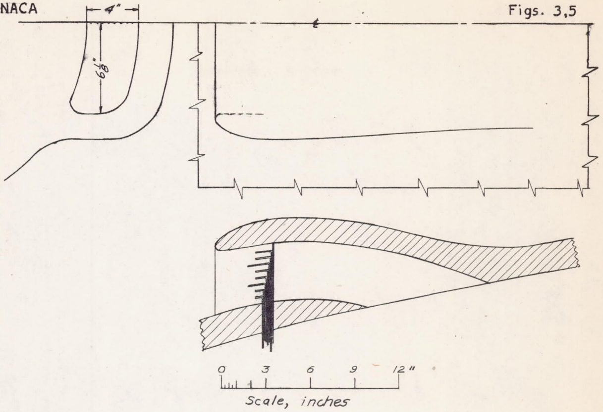
Figure 3.- Scoop A-1.
