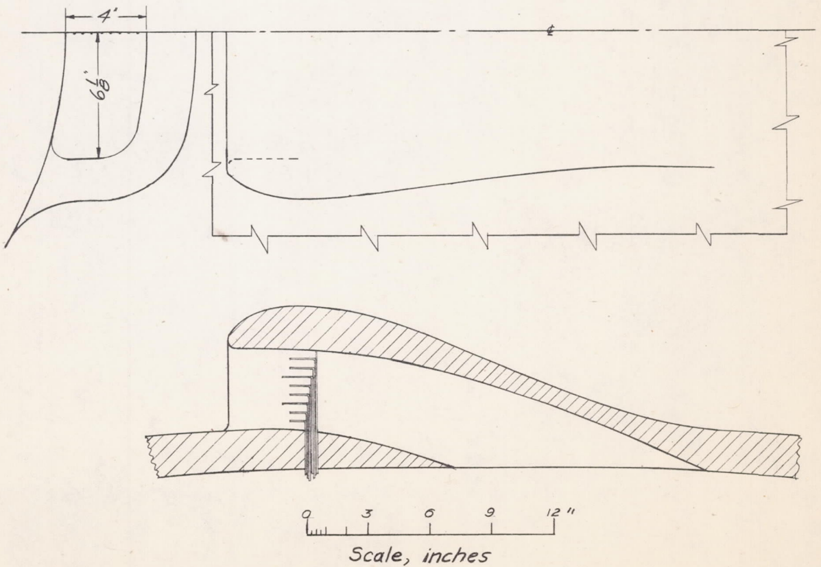
Figure 5.- Scoop B-1.
