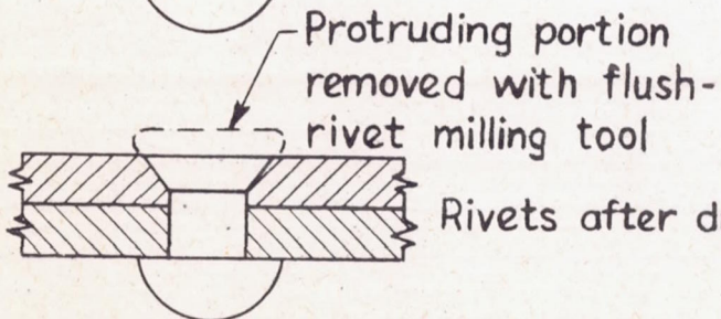
(a) NACA flush rivet.
